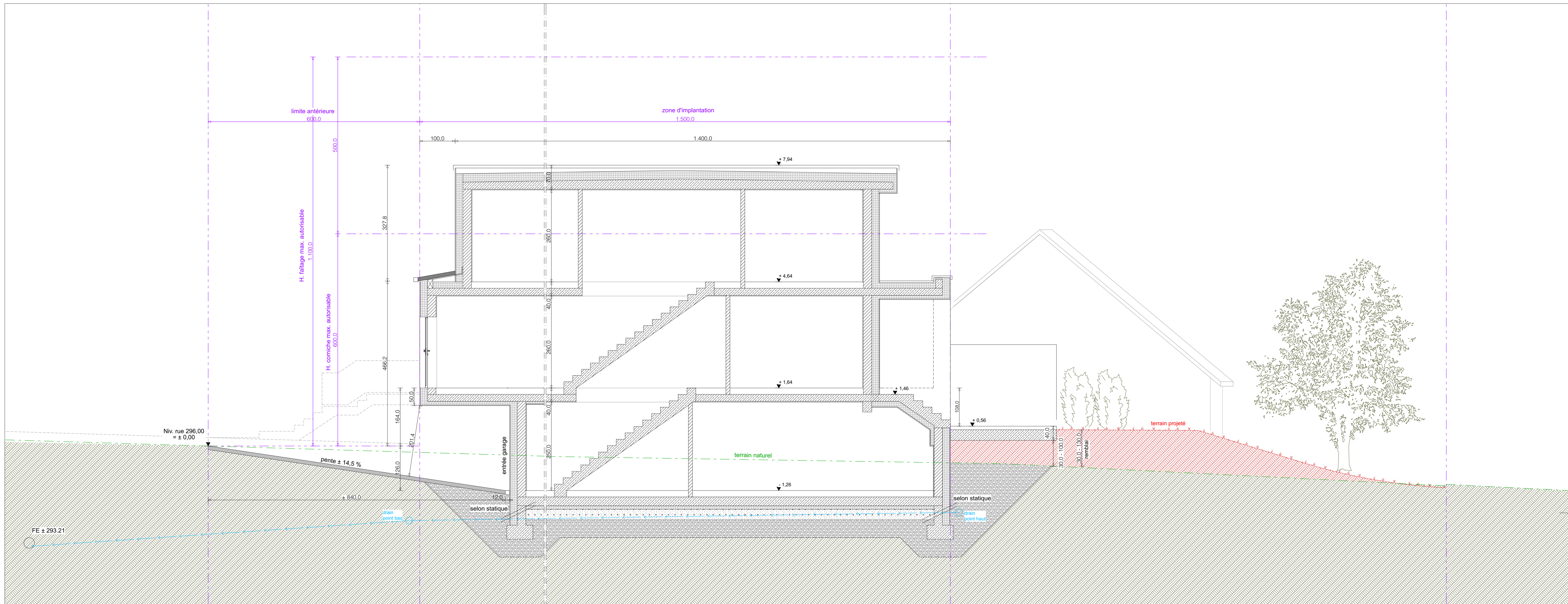
COUPE A (LONGITUDINALE)
